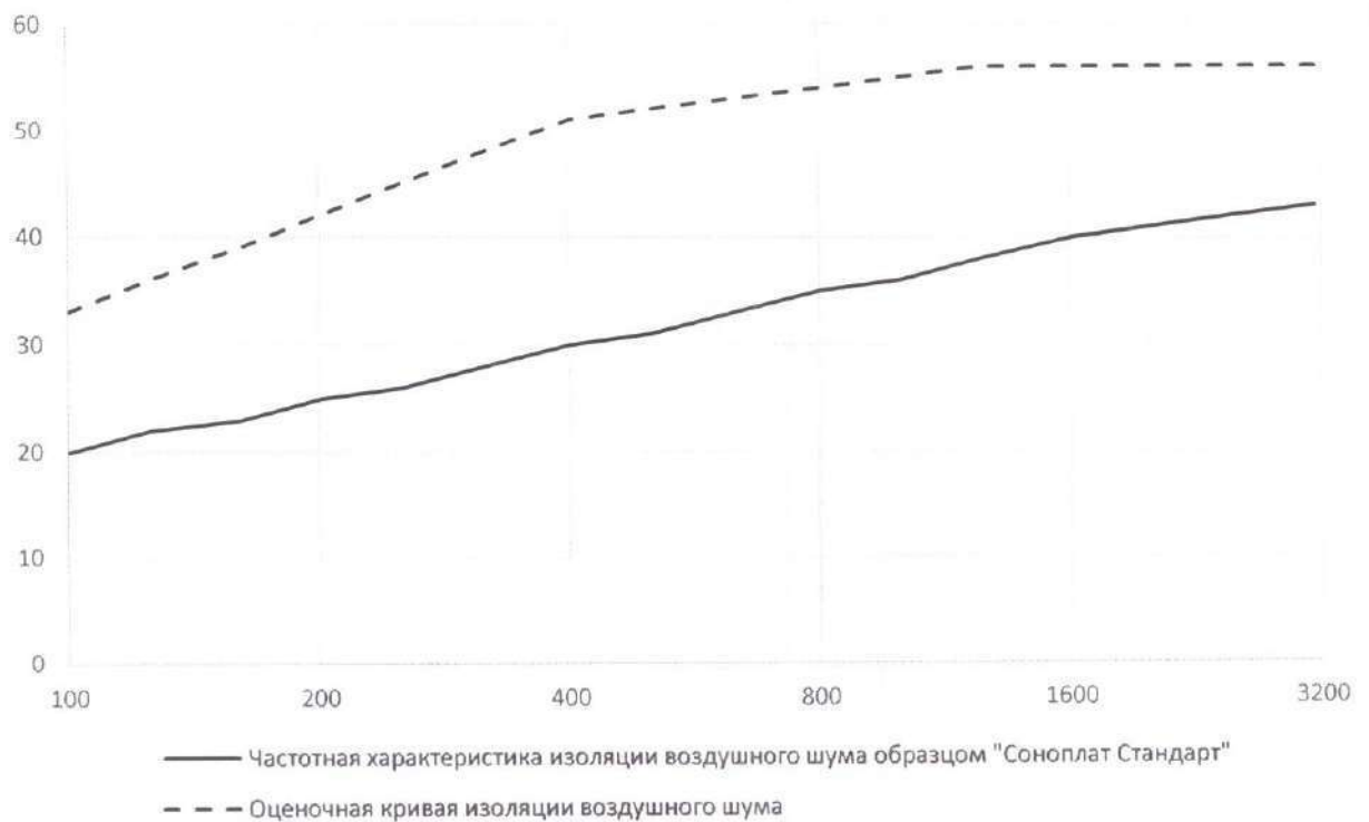
Рисунок 1. График частотной характеристики изоляции воздушного шума образцом материала «Соноплат Стандарт»
